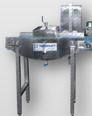
Chladiaci dopravník
